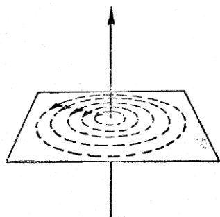
Fig. 2 - Spettro di Arago del campo magnetico concatenato ad un filo percorso da corrente elettrica.
