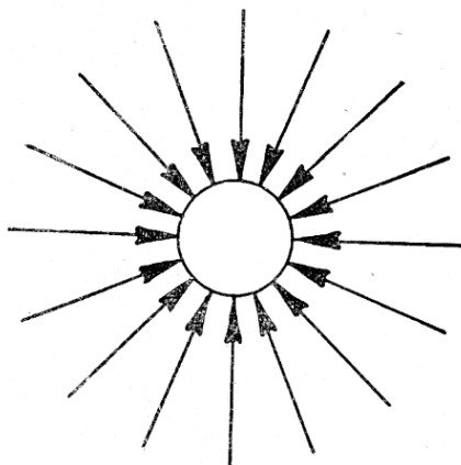
Fig. 1 - Grafico del campo di gravitazione astronomica e del campo di attrazione elettrica del nucleo atomico.
