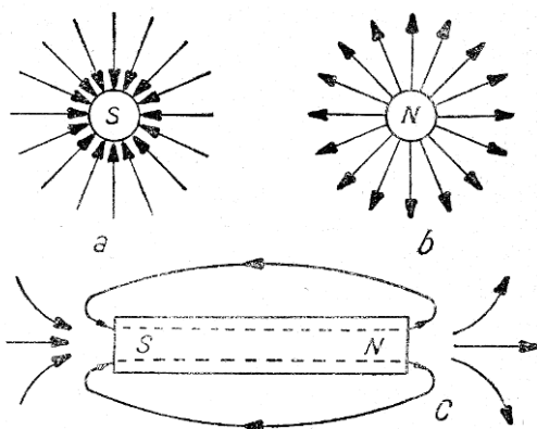
Fig. 3 - Spettri di Arago del campo magnetico di una calamita naturale. a) - b) prospetti polari - c) prospetto longitudinale.
